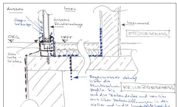
Abb. 2: Skizze zur Wegführung der eindringenden Regenwassermengen
