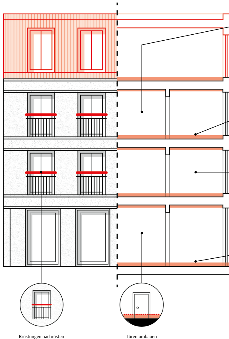
Abb. 8: Bauliche Folgewirkungen im Bestand
